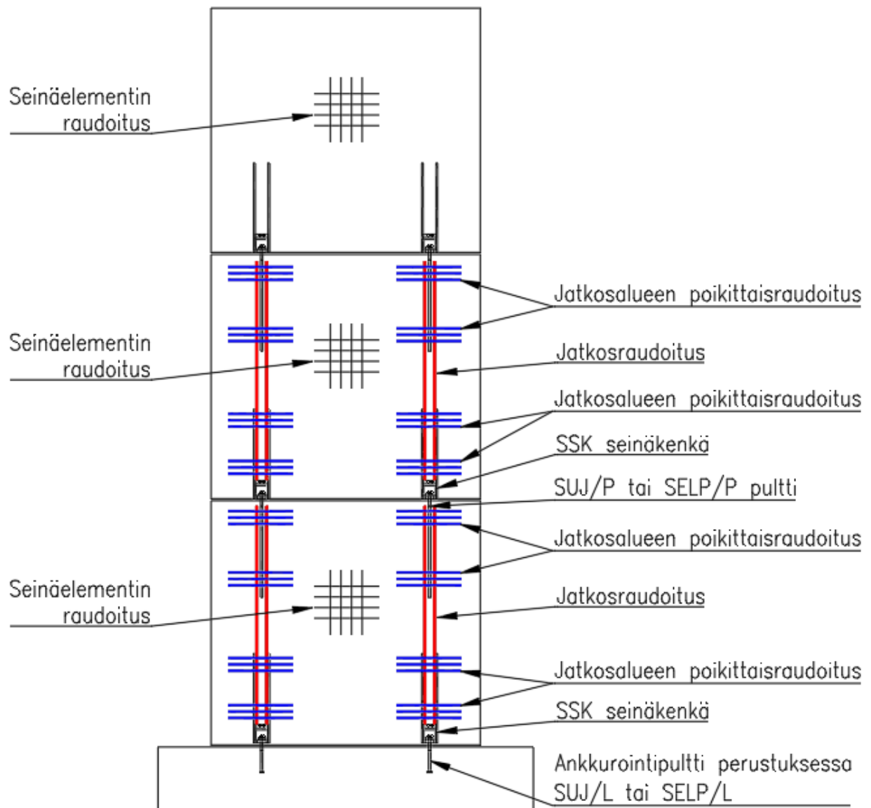
Kuva 5. Seinäelementin raudoitus
