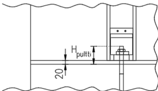
Kuva 8. Pulttien korkeusasema
