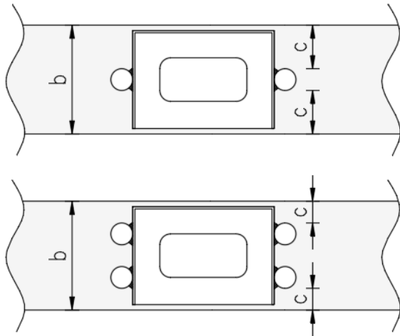
Kuva 4. SSK-seinäkenkien seinäelementin paksuus ja betonipeite
