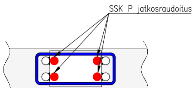
Kuva 6. SSK-seinäkenkien jatkosraudoituksen sijoitus seinäkenkien tartuntojen viereen
