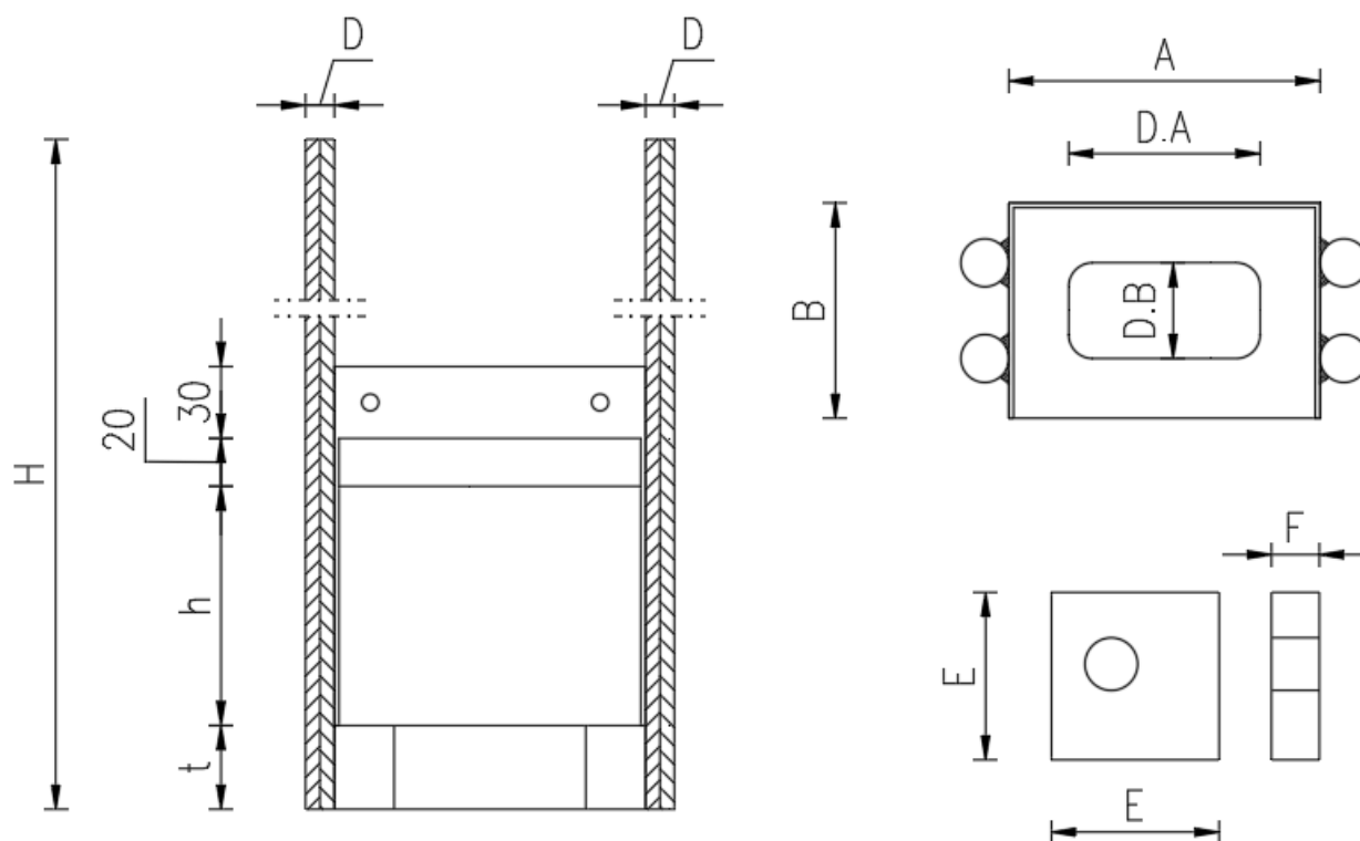
Kuva 2. SSK P -seinäkenkien mitat
