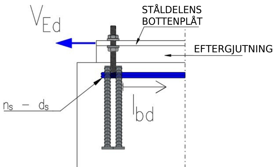
Figur 12. Skärkraftsarmering för SELP-grundbultar
