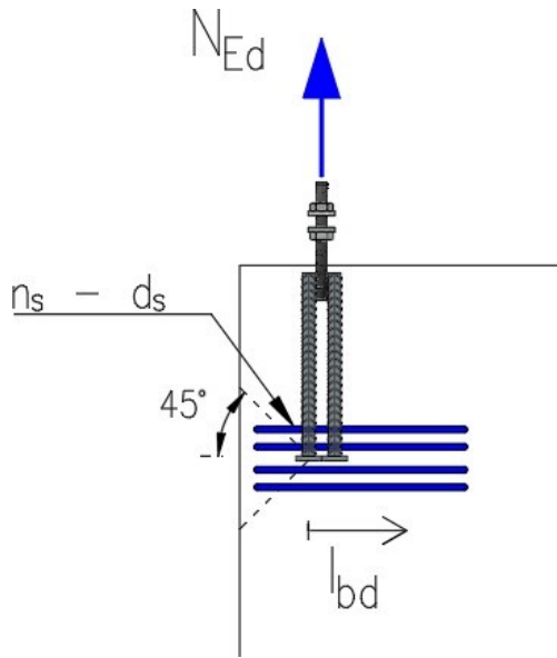
Figur 10. SELP/L-grundbultars kantbrottarmering
