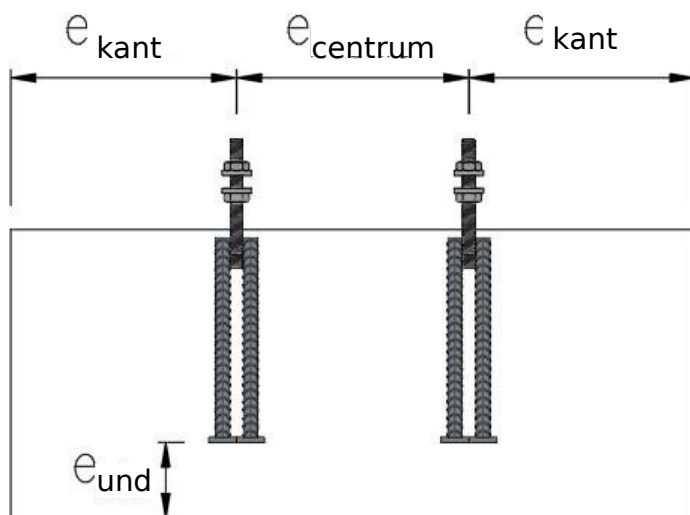
Figur 5. SELP/L-grundbultarnas minimiavstånd
