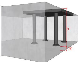
Figur 3 Minsta kantavstånd mellan studs och betongyta.
