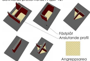
Figur 12 Definition av angreppsarea.
