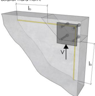
Figur 14 Fästplåt nära hörn.
