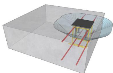
Figur 5 Utformning av tilläggsarmering. c_{min} i Figur 5 motsvarar c_1 i Tabell 6.
