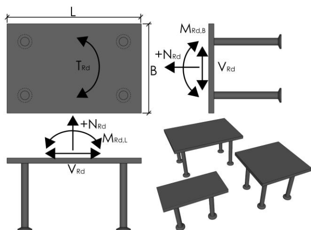
Figur 2 Beteckningar på kapaciteter.
