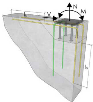
Figur 16 Fästplåt i vägg.
