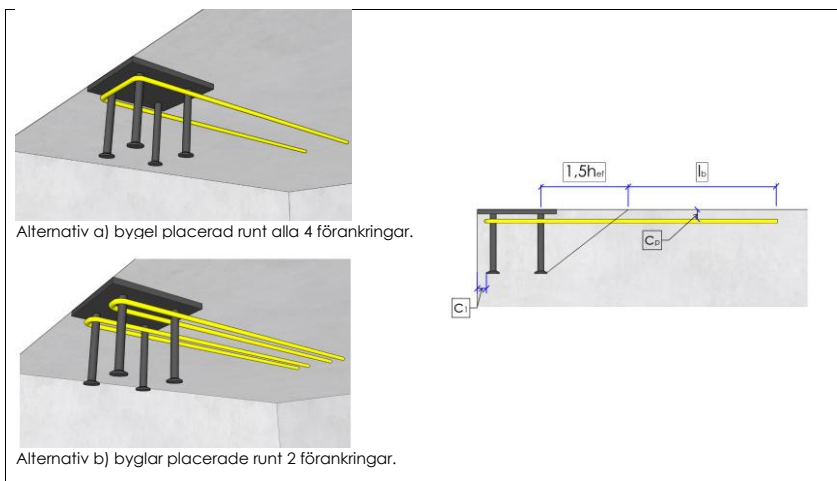
Figur 10 Tilläggsarmering för betongkantbrott.
