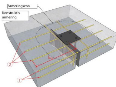
Figur 7 Armering för spräckning. Betongkvalitet C25/30-C40/50.
