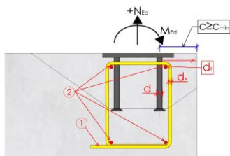
Figur 5 Utformning av tilläggsarmering. c_{min} i Figur 5 motsvarar c_1 i Tabell 6.
