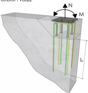
Figur 15 Fästplåt i vägg.
