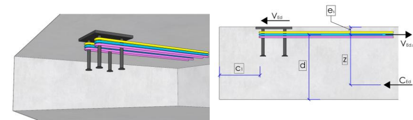
Figur 11 Tillskott av dragkraft i tilläggsarmering.
