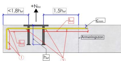
Figur 7 Armering för spräckning. Betongkvalitet C25/30-C40/50.
