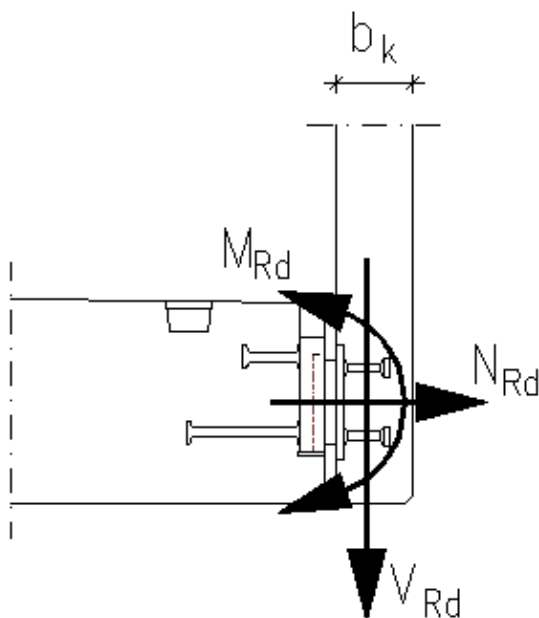
Kuva 5. Voimien ja kestävyyslaskennan merkinnät PL-kaideliitoksessa
