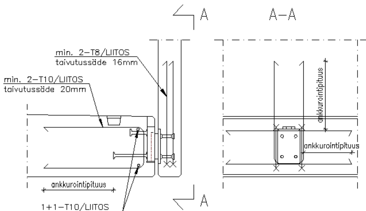
Kuva 8. PL-kaideliitoksen vaatima lisäraudoitus
