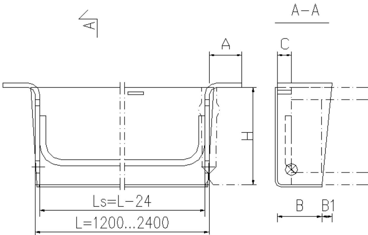
Kuva 1. PBOK-ontelolaattakannakkeen mitat
