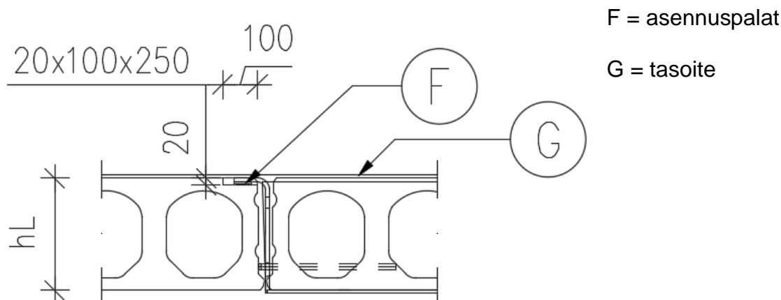
Kuva 4. PBOK-ontelolaattakannake madalletulla tukiosalla
