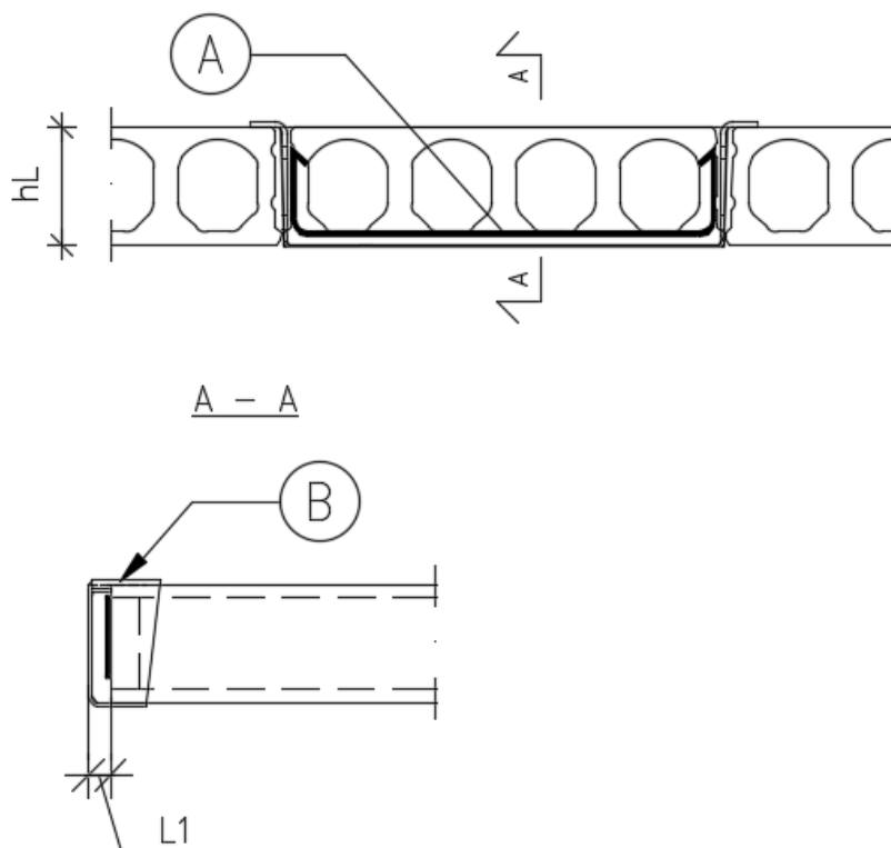
Kuva 2. Mitta L1 ja paloteräs
