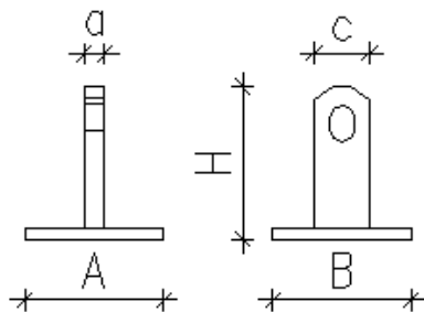
Kuva 1. RR-nostoankkurit, tyypit
